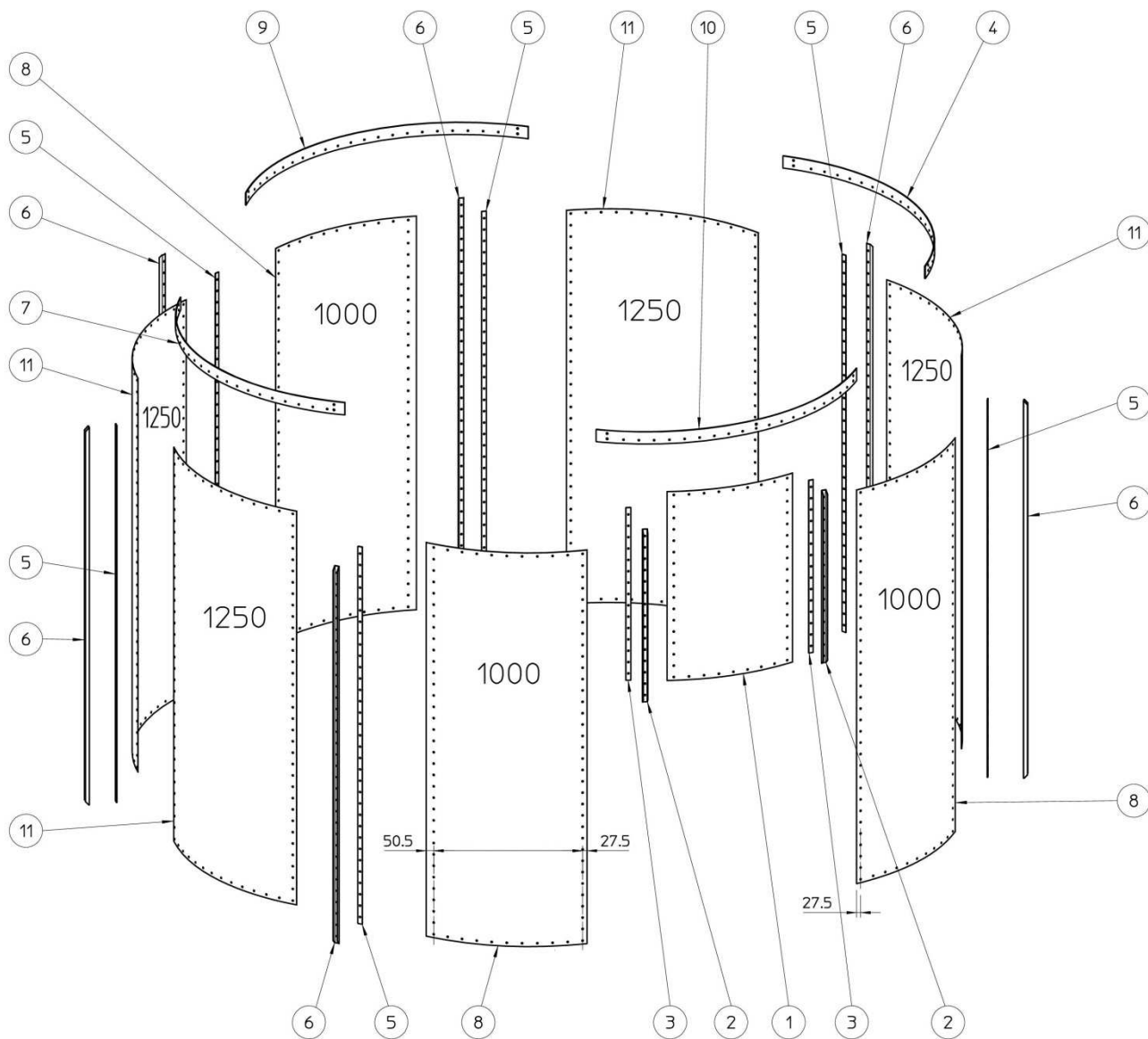
FIG.49 Cilindro di base – Base cylinder
