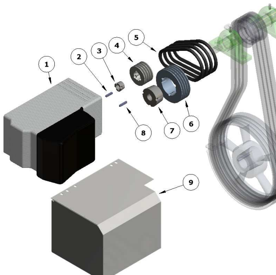
FIG. 5 Trasmissione del generatore – Generator transmission
