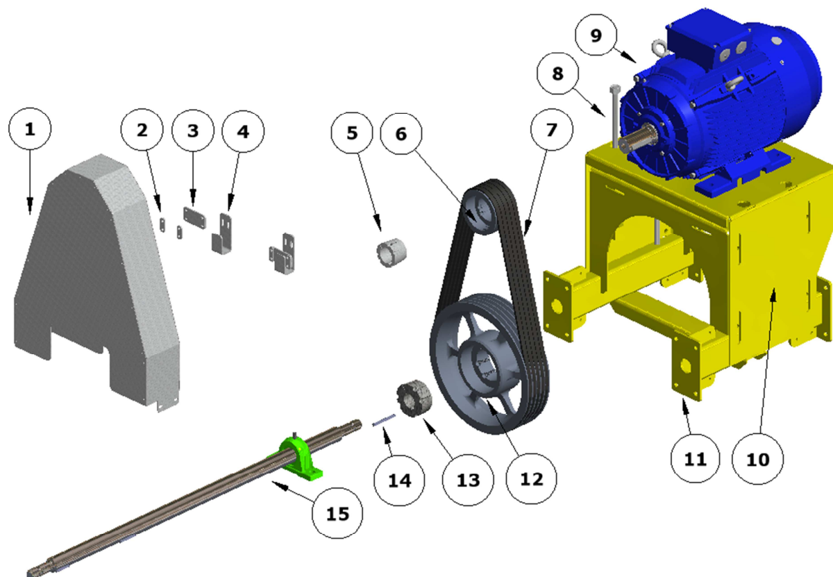
FIG. 9 Aggiunta trasmissione PTO+1 ME - PTO+1ME Transmission
