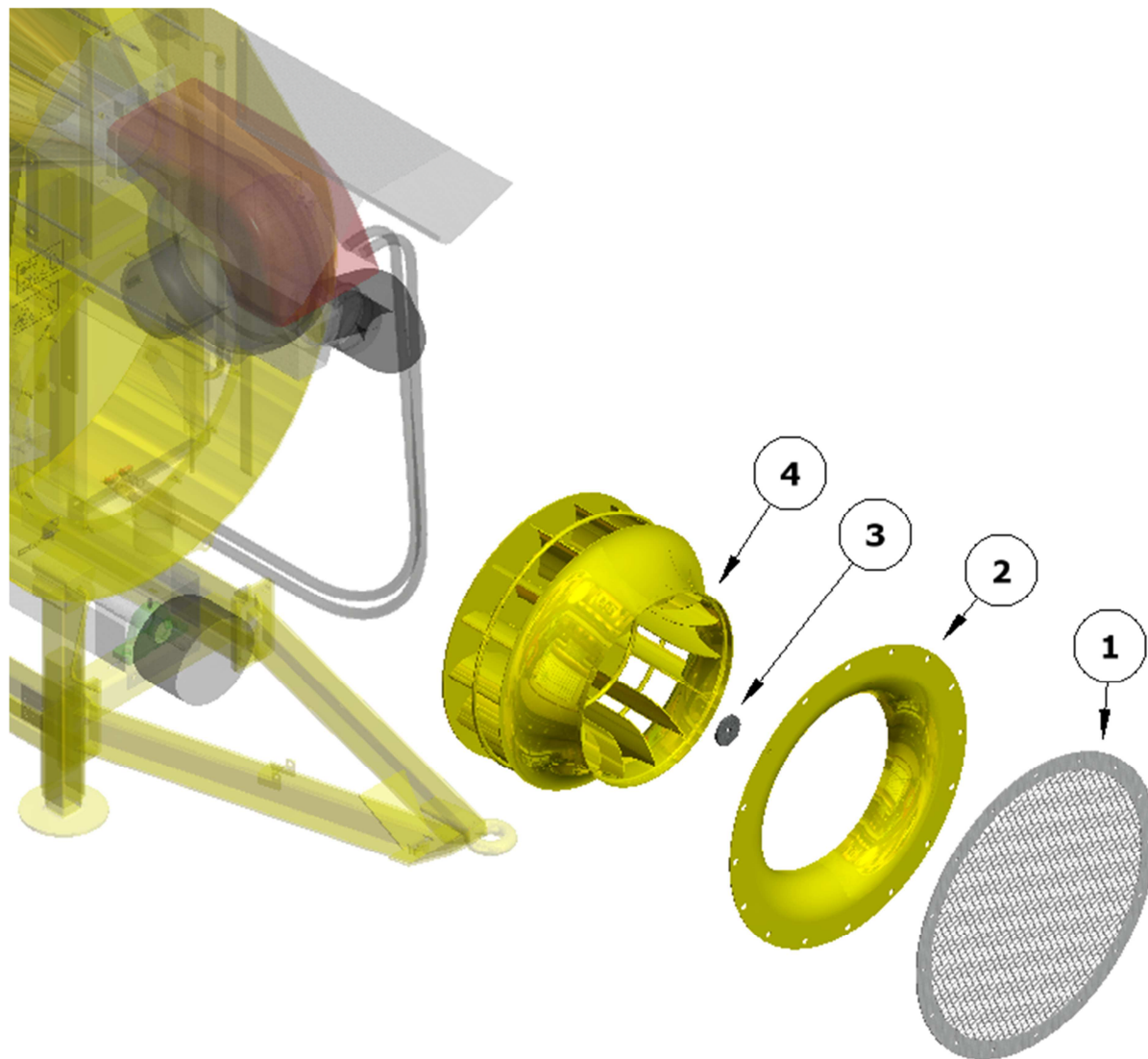
FIG. 16 Ventilatore – Fan
