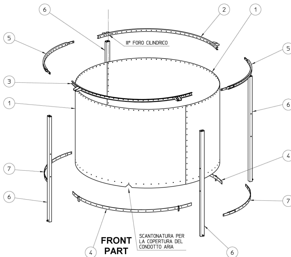
FIG.50 TELESCOPICO - Telescopic Configurazione a richiesta del cliente – Configuration on request by customer
