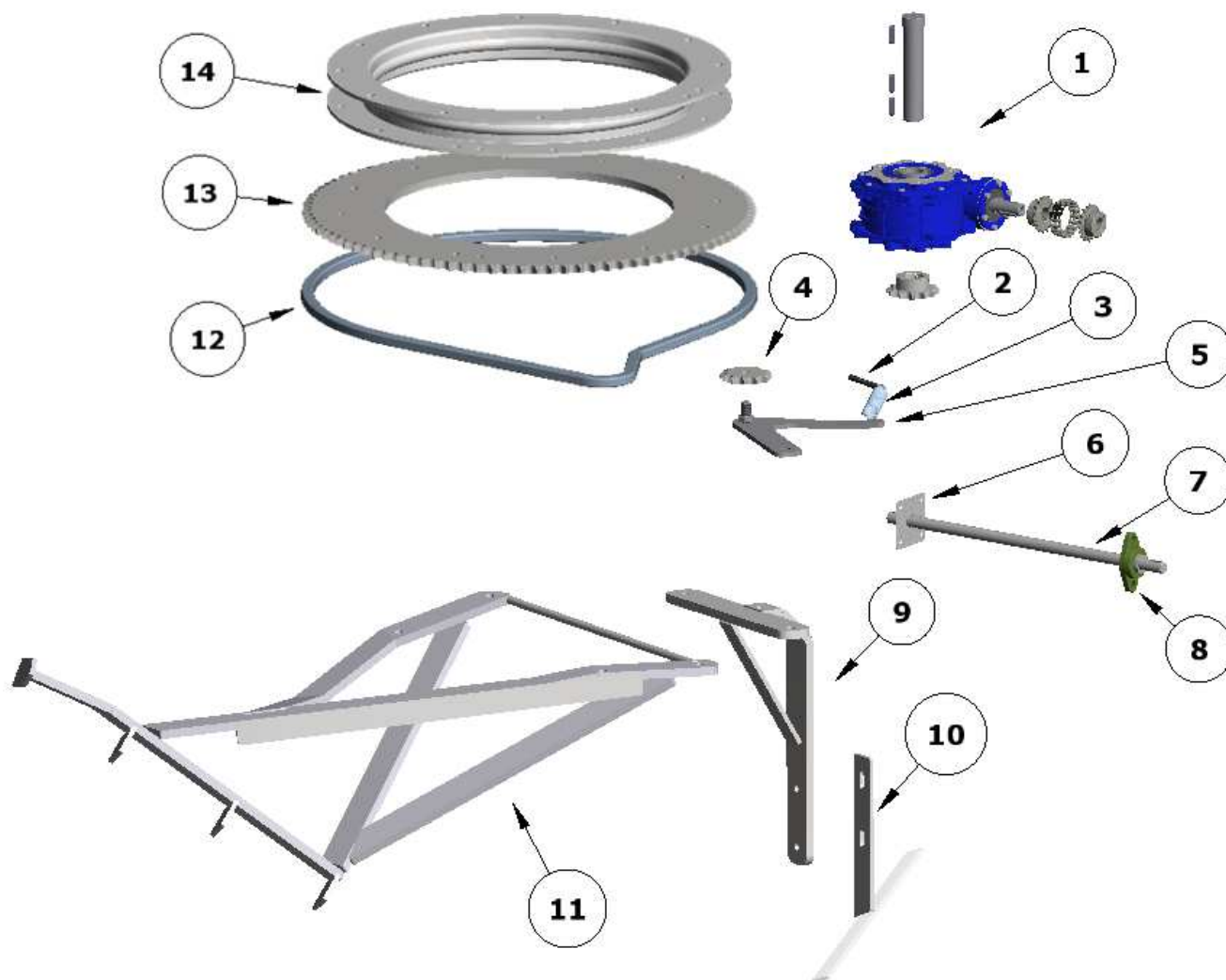
FIG. 29 Trasmissione miscelatore – Scraper transmission
