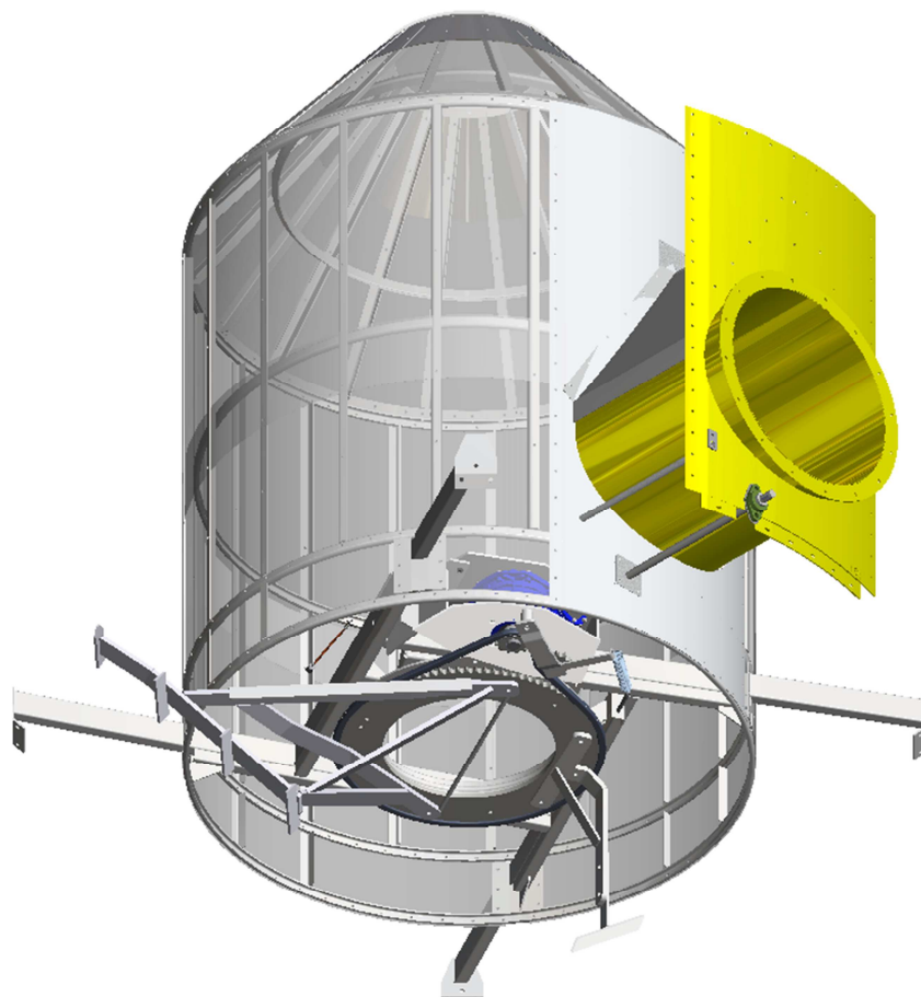
Cesto interno - Plenum chamber o internal cylinder
