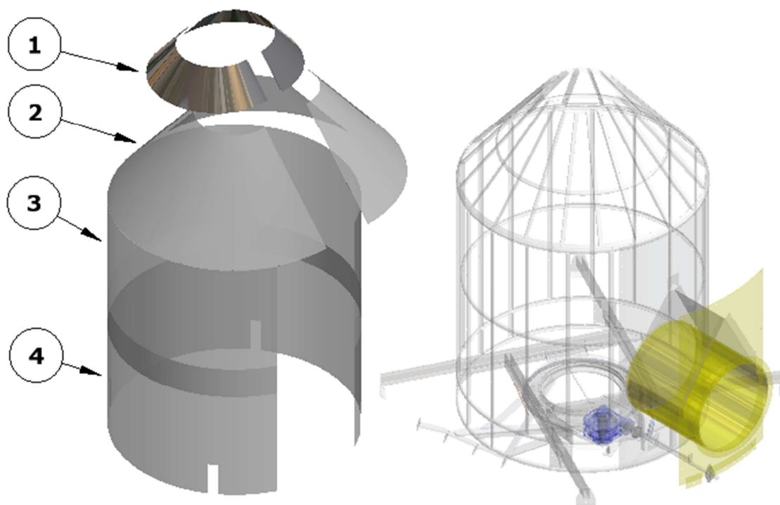
FIG.51 CESTO INTERNO – Plenum chamber Configurazione a richiesta del cliente – Configuration on request by customer
