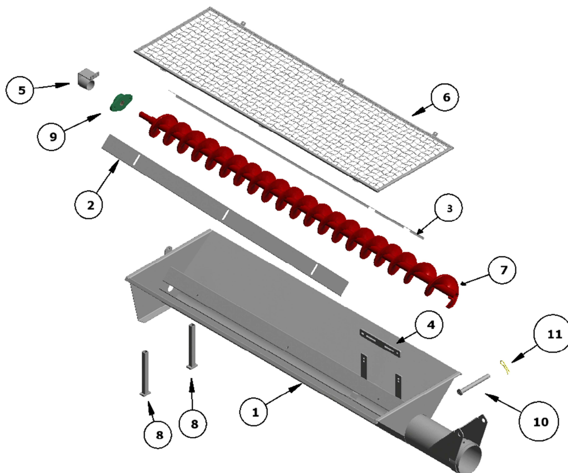
FIG. 21 Tramoggia di carico UK – Loading hopper UK
