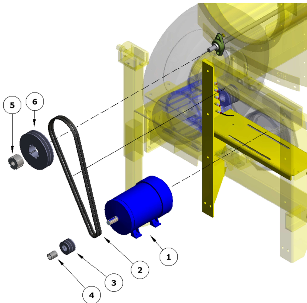
FIG. 27 Trasmissione elettrica miscelatore – Electric transmission for scraper
