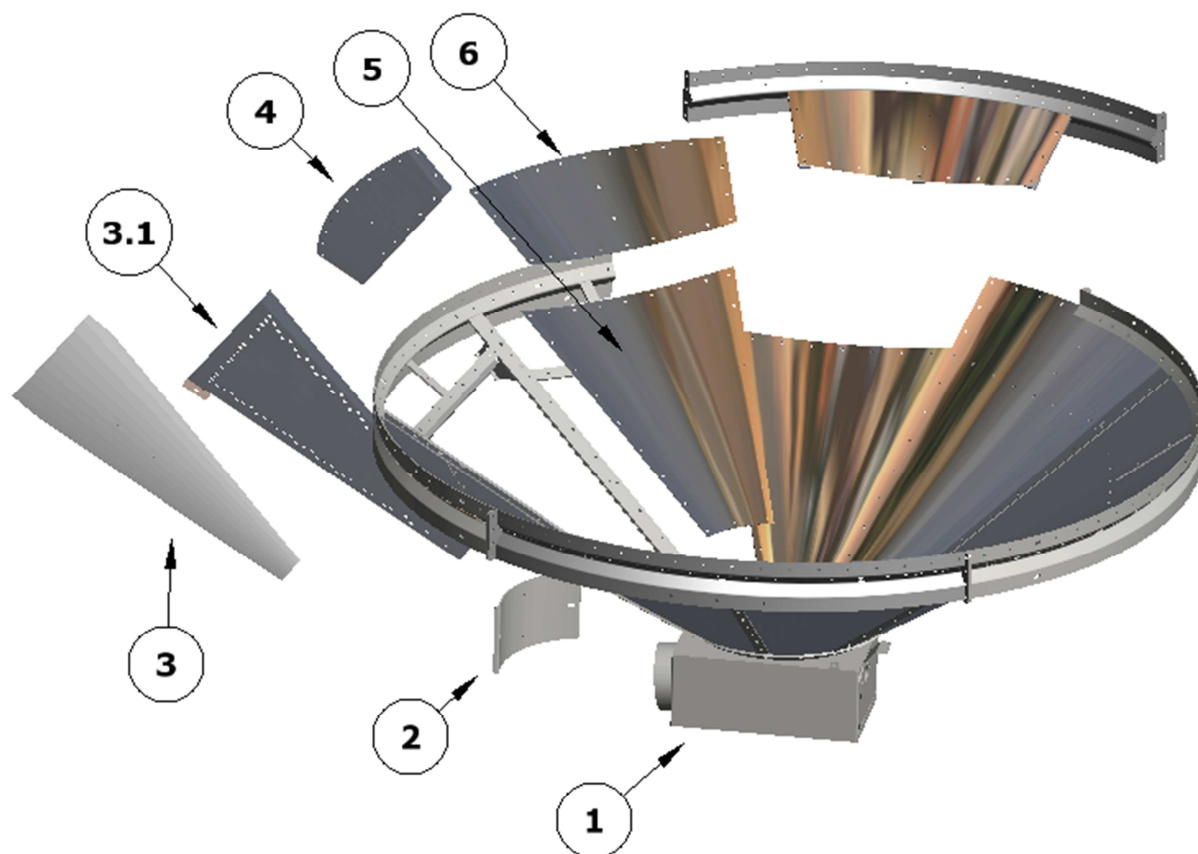
FIG.48 Cono di base – Bottom cone Configurazione a richiesta del cliente – Configuration on request by customer
