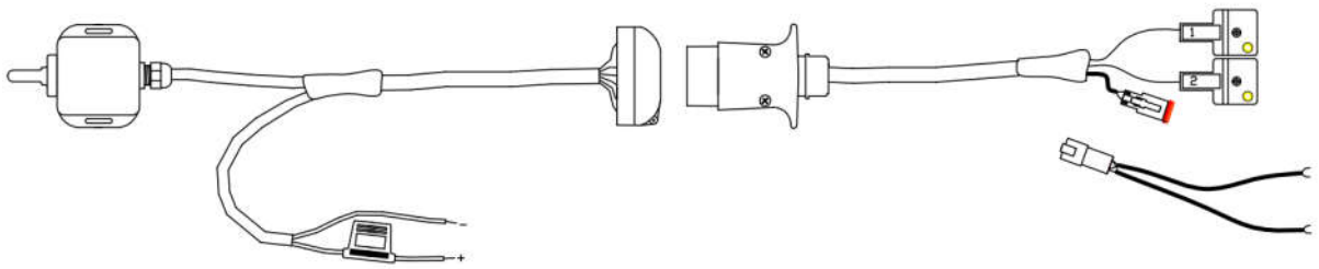
Tegning 1. U-fresens strømledning
