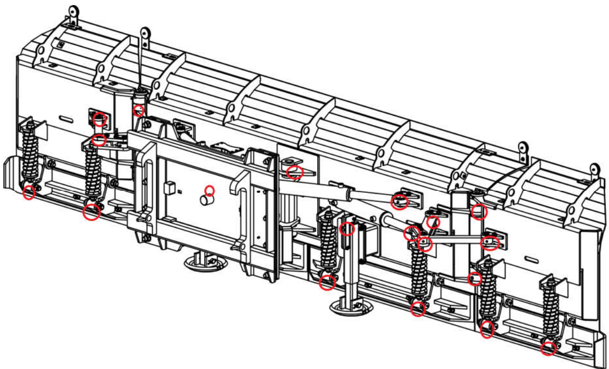
Tegning 4. Plassering av smørenipler
